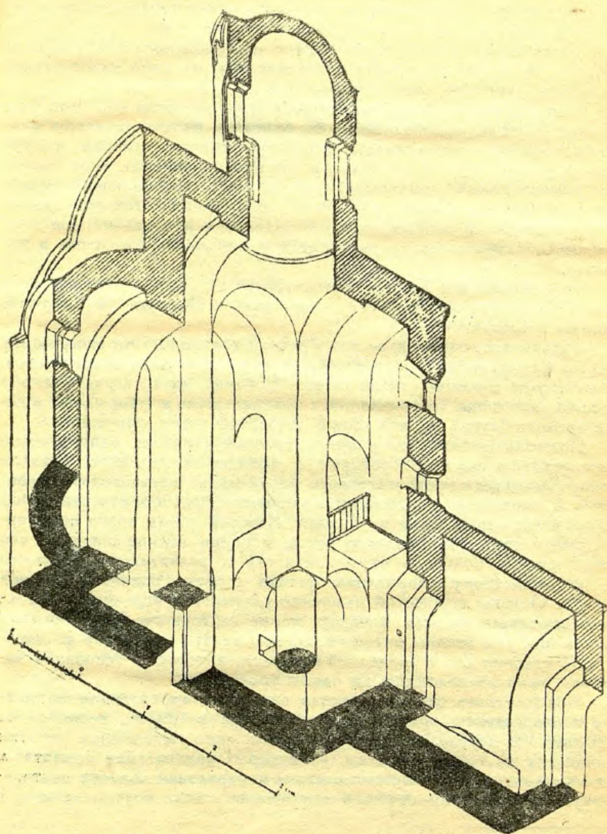
Рис. 2. Разрез конструкции Вологовской ц. (масштаб в саженьях).
